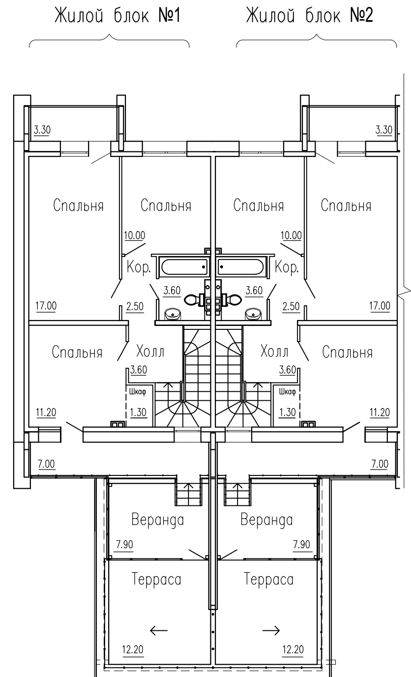
План 2 этажа
