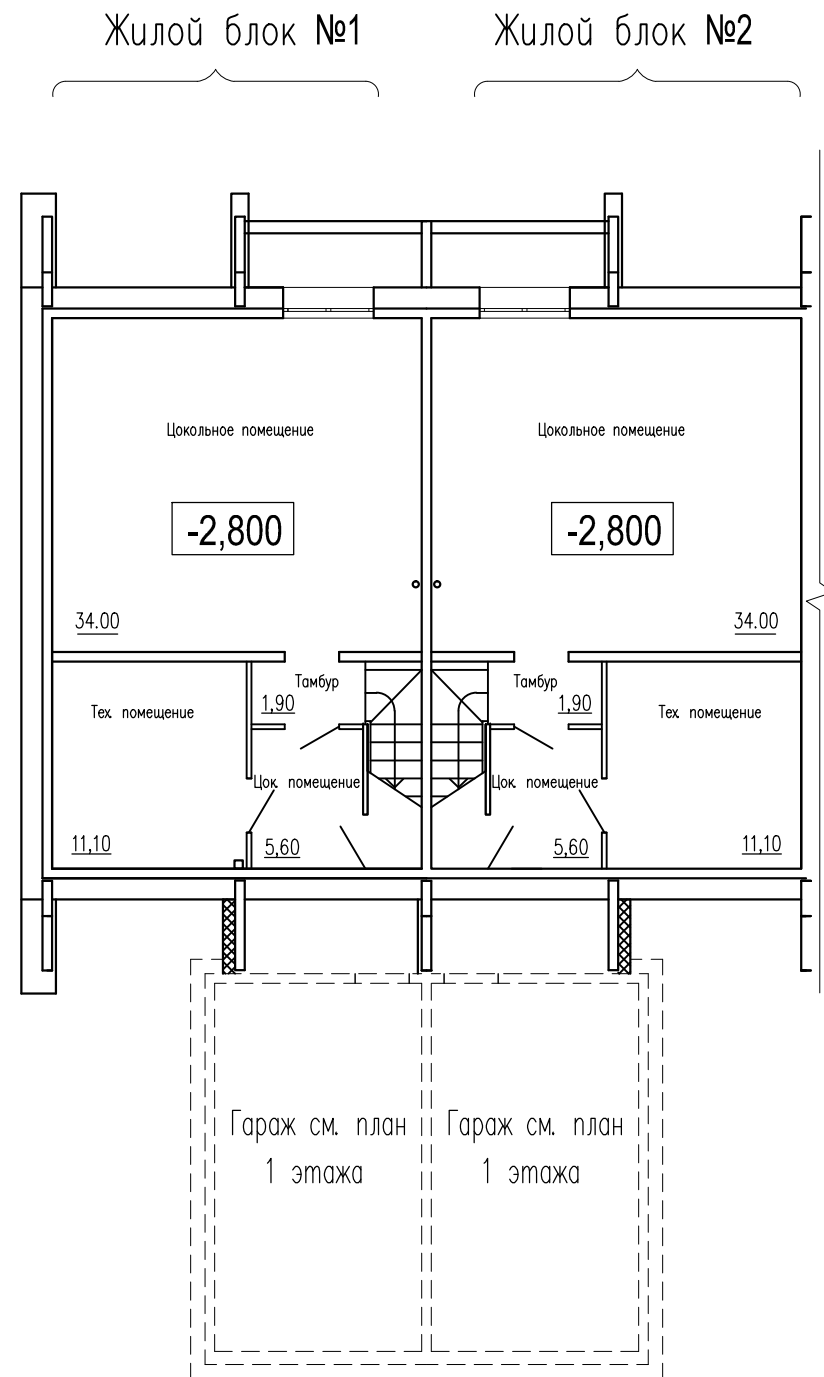
План на отм.-2.800
