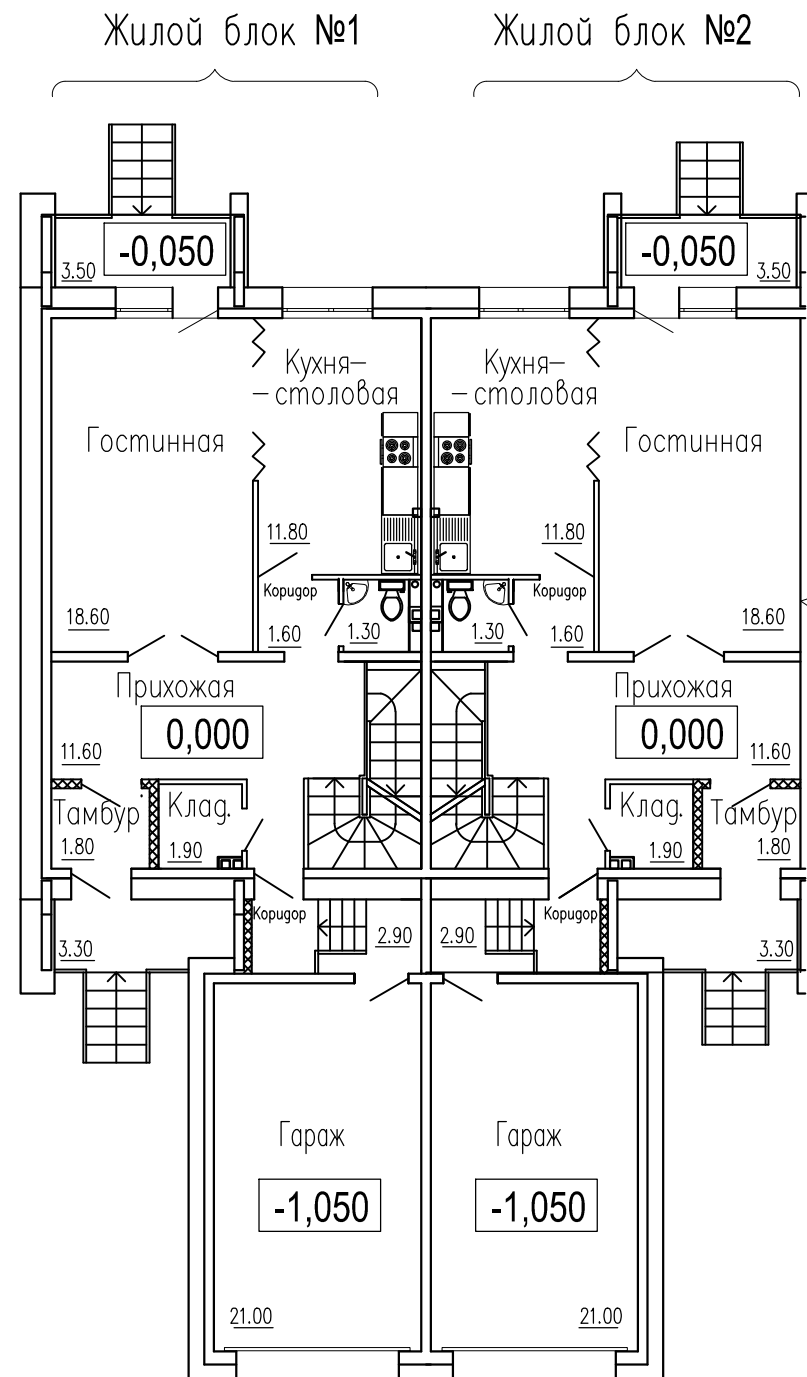
План 1 этажа
