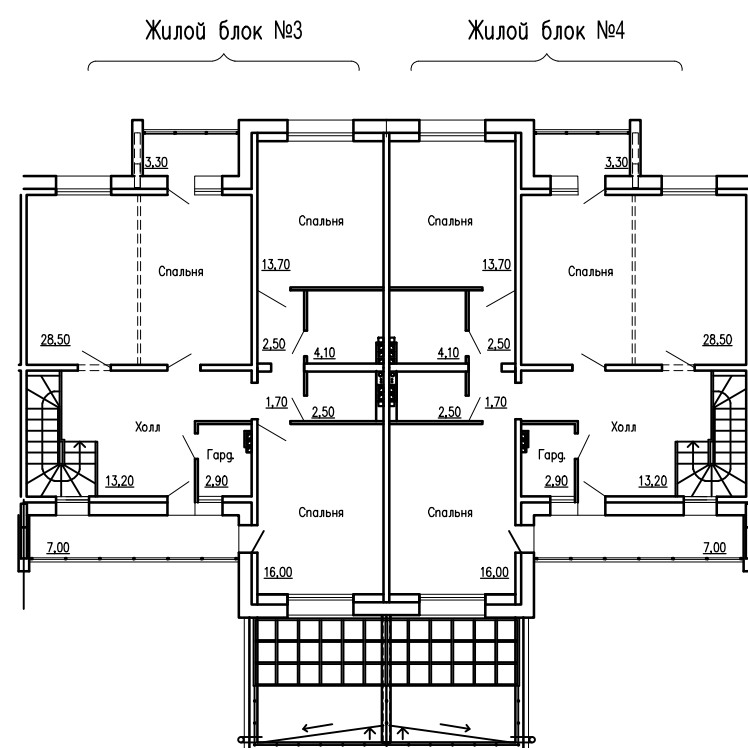
План 2 этажа
