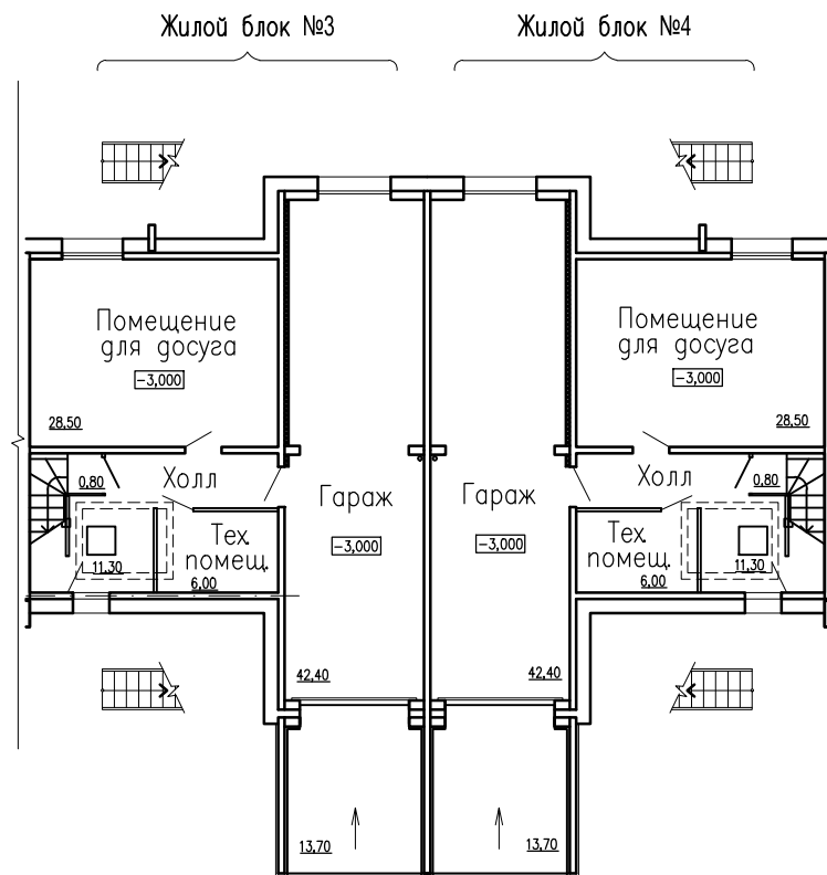
План 1 этажа
