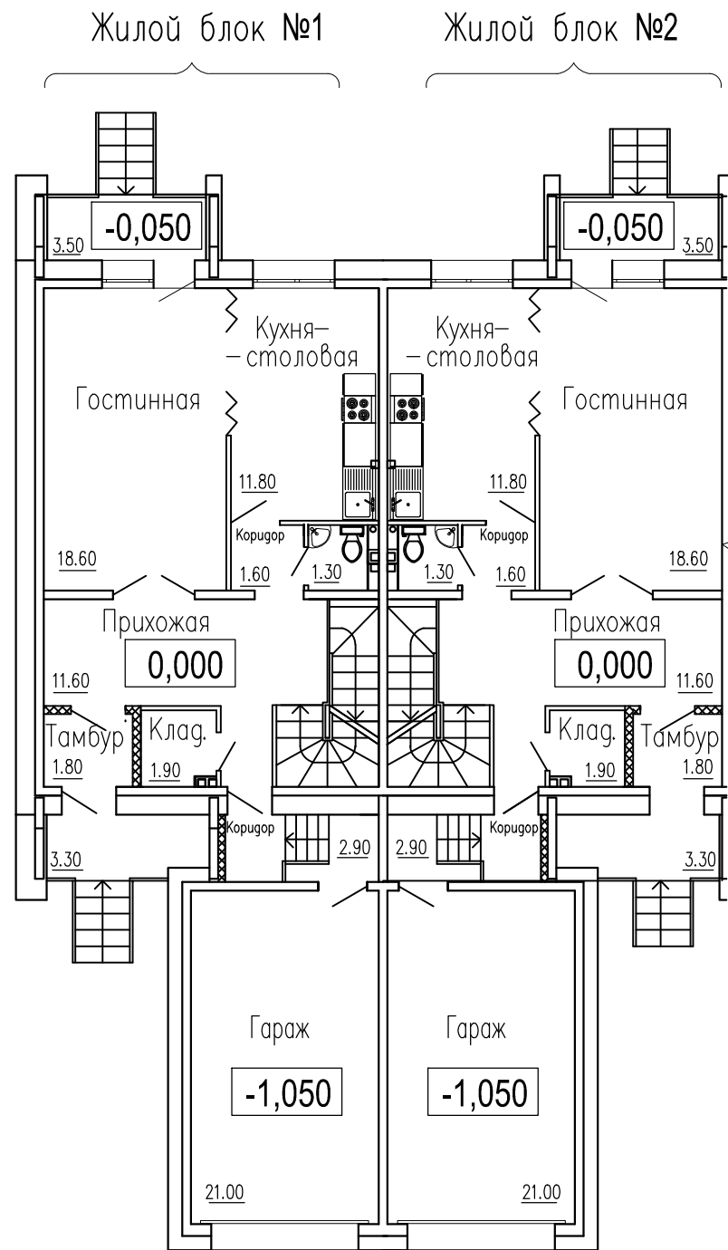
План 1 этажа
