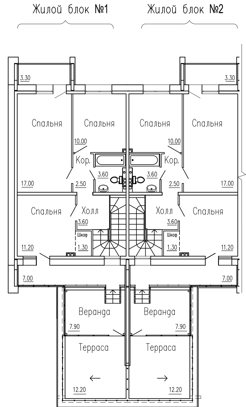
План 2 этажа
