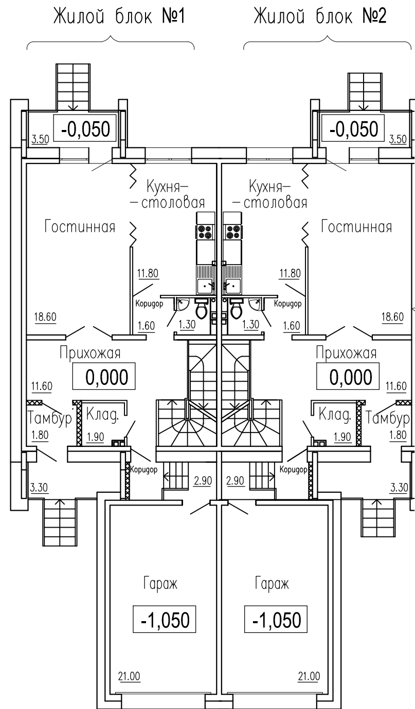
План 1 этажа
